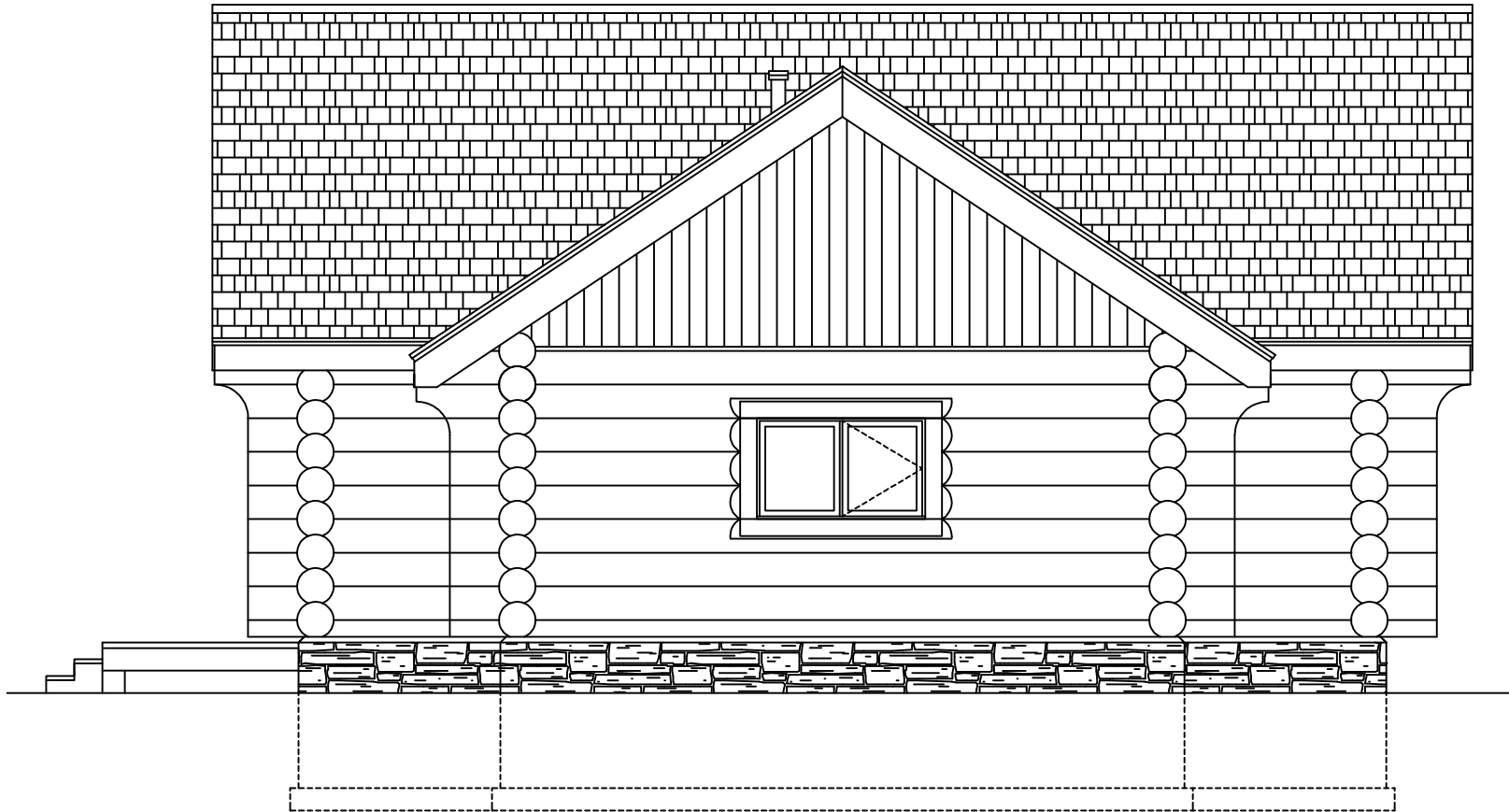
Right Elevation
